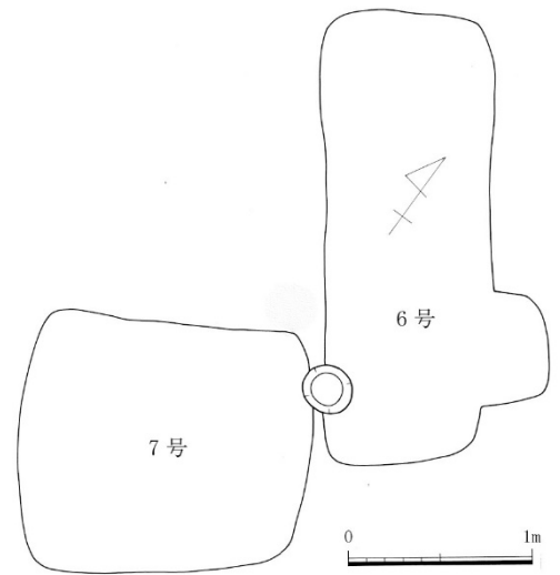
图 3-12 船原古墳 6 号・7 号 土坑実測図
