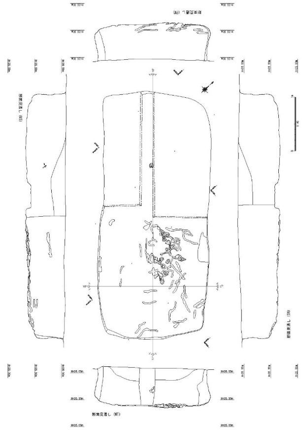
图 3-8 船原古墳 2 号土坑遺構図
