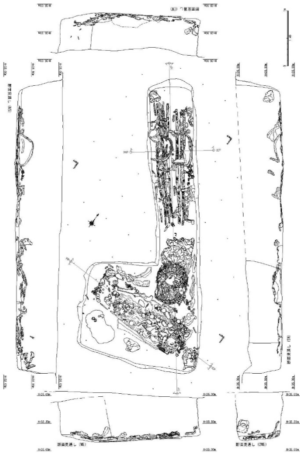
图 3-7 船原古墳 1 号土坑遺構図
