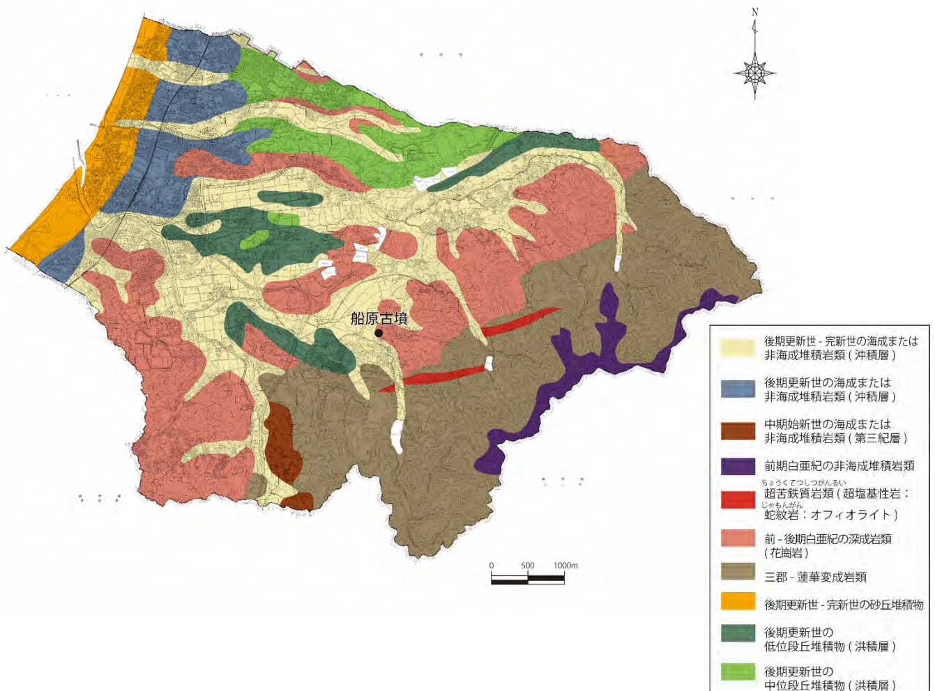
図 2-3 古賀市地質概要図（産総研地質調査総合センター，20 万分の 1 日本シームレス地質図より）
