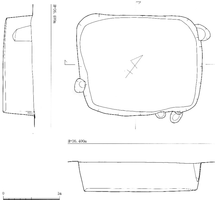
图 3-10 船原古墳 4 号土坑実測図
